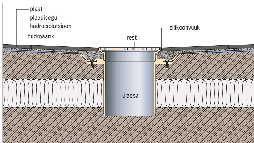
Paigaldusskeem
